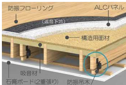
●床遮音〈ノイズレスシステム〉
